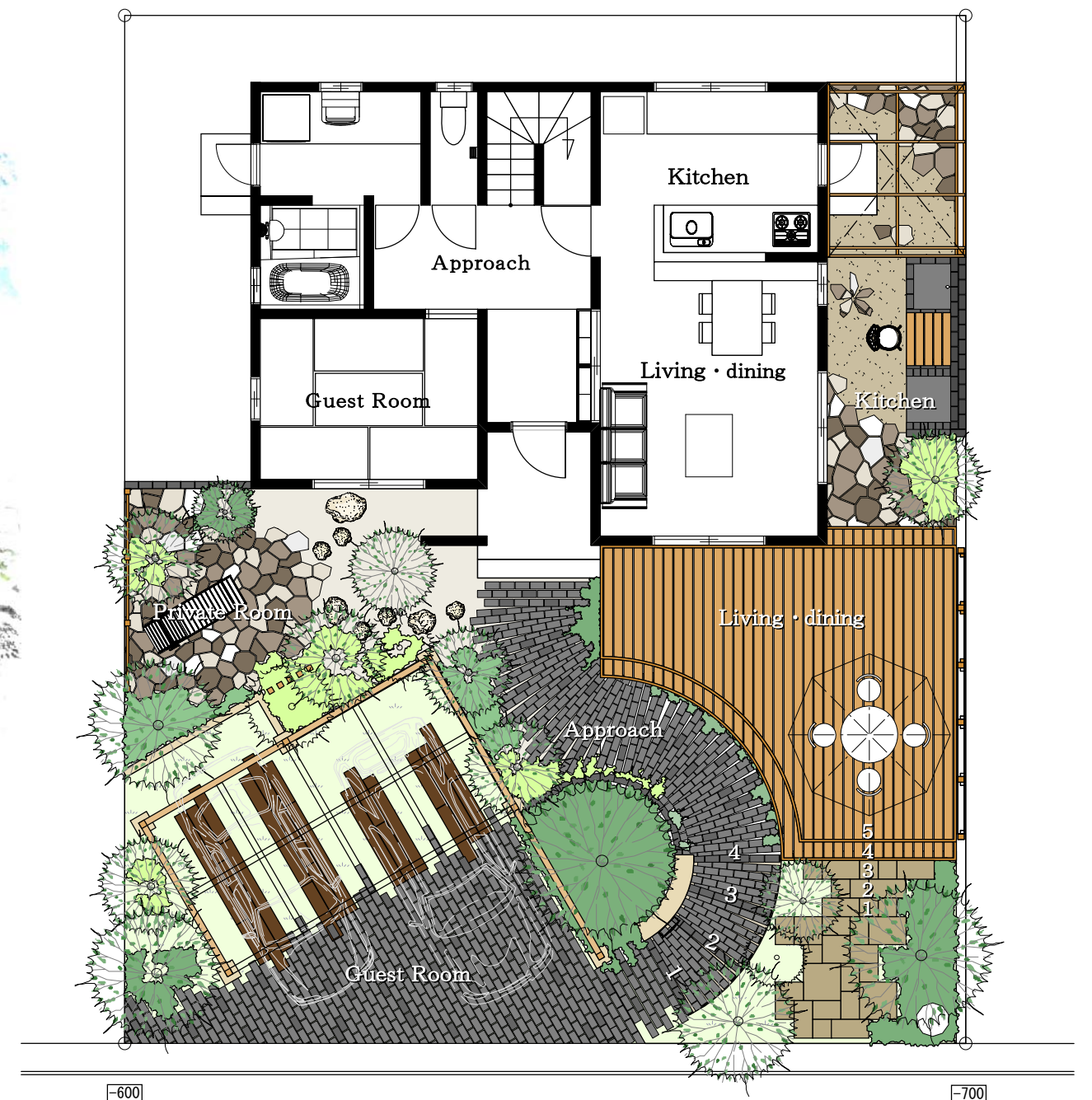
1F Plan=1 : 100
