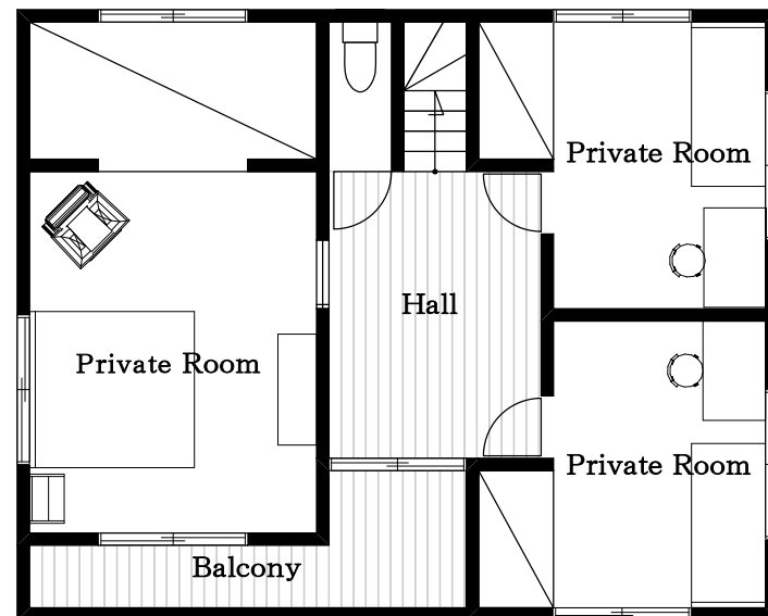
2F Plan=1 : 100
